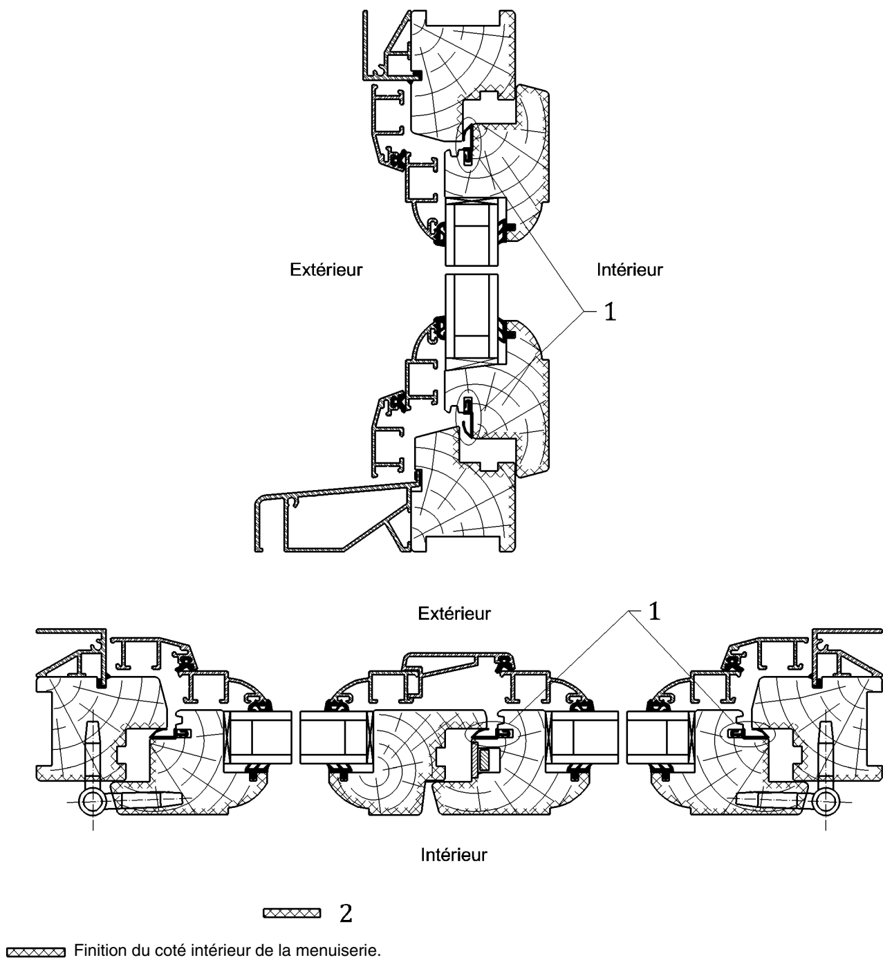
Figure B.3 — Cas d'une menuiserie bois-alu
