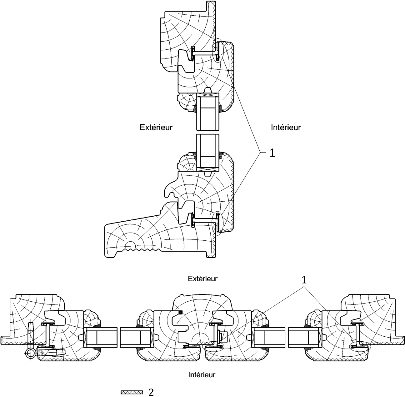
Figure B.2 — Cas d'une menuiserie bois
